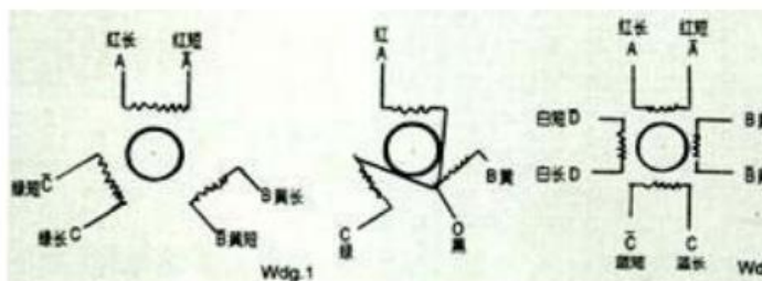
接线图1
